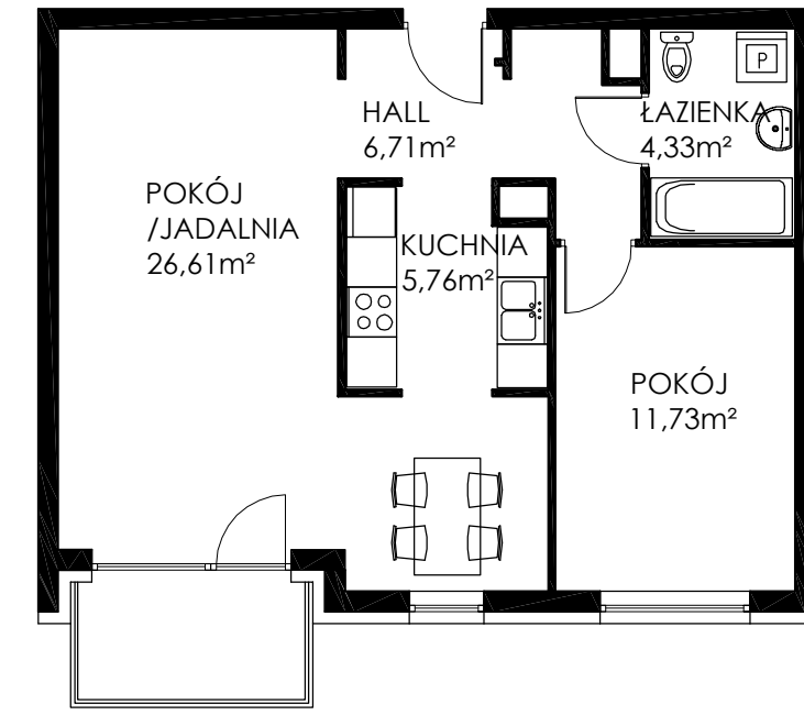
2 POKOJE + KUCHNIA MIESZKANIA NR: 38,39,40,41, 44,45,46,47 powierzchnia - 55,14 m 2 ilość na piętrze III - 8
