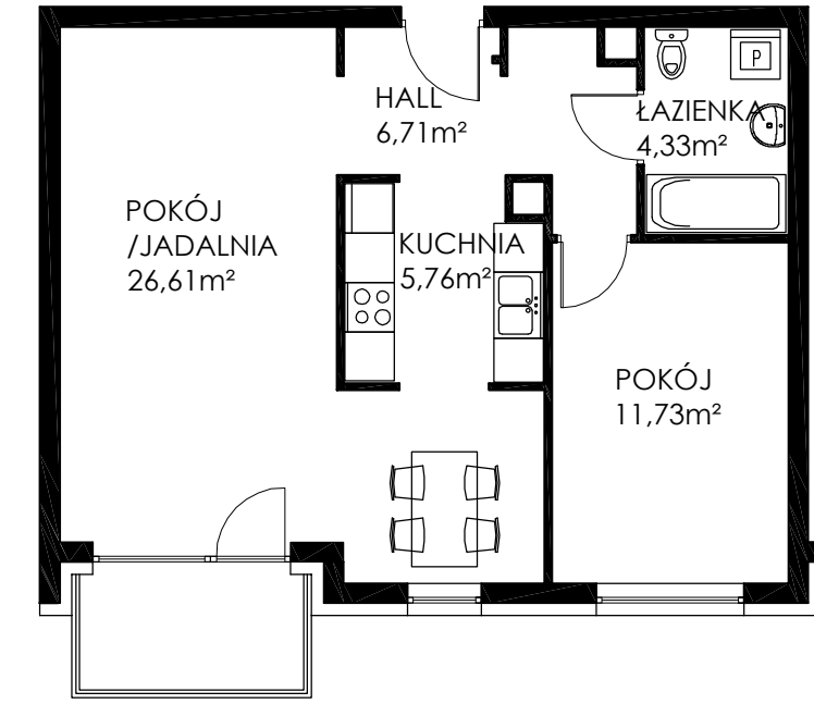
2 POKOJE+KUCHNIA MIESZKANIA NR: 2,3,4,5,8,9,10,11 powierzchnia - 55,14 m 2 ilość na parterze - 8
