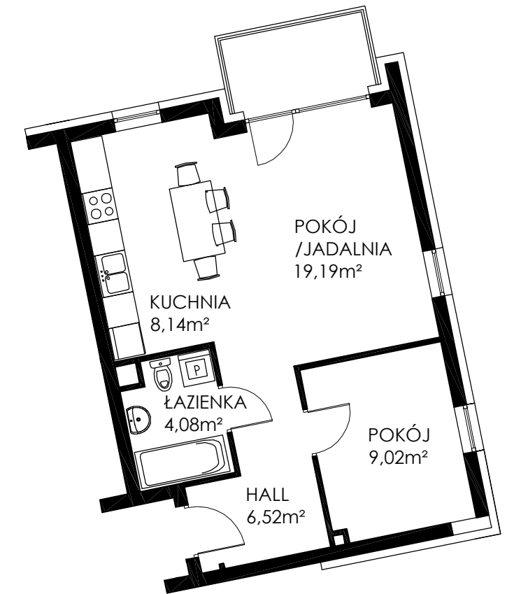
2 POKOJE+KUCHNIA MIESZKANIE NR: 12 powierzchnia - 47,12 m 2 ilość na parterze - 1
